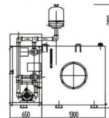
一种可移动式油污净化系统 专利号:ZL2020200411688
